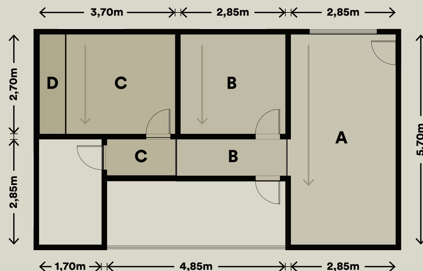
PLANTA BAIXA
