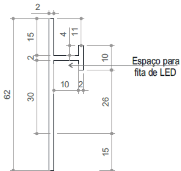
Figura 4 - Espaçamento de 10 mm se faz necessário, para colar o verso da fita de LED, conforme indicação da seta.
