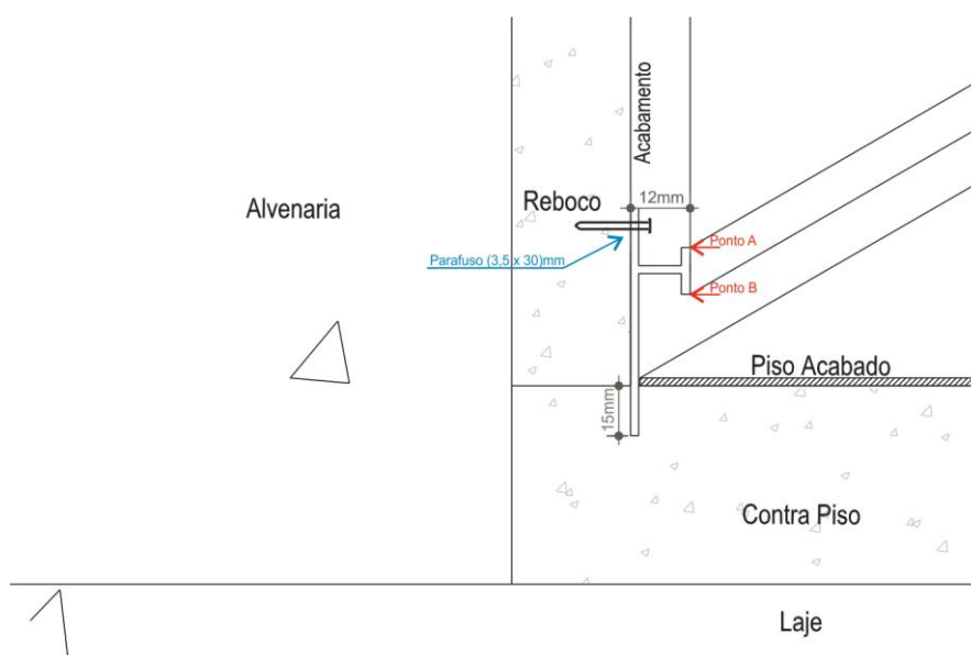
Figura 2 – Vista em corte da instalação.
