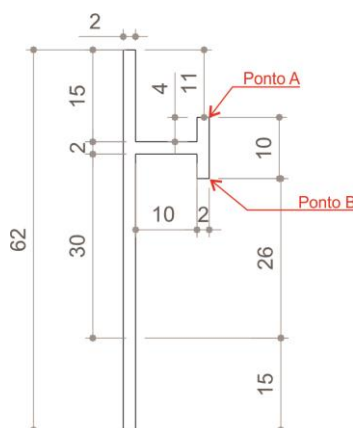
Figura 1 – Dimensões em milímetros
