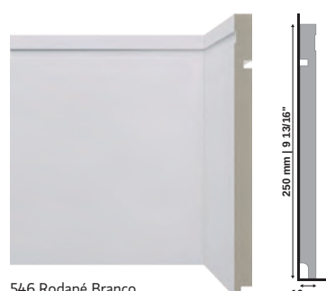
546 Rodapé Branco White Wall Base | Zócalo Blanco
