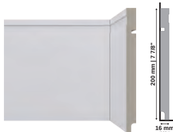
505 Rodapé Branco White Wall Base | Zócalo Blanco
